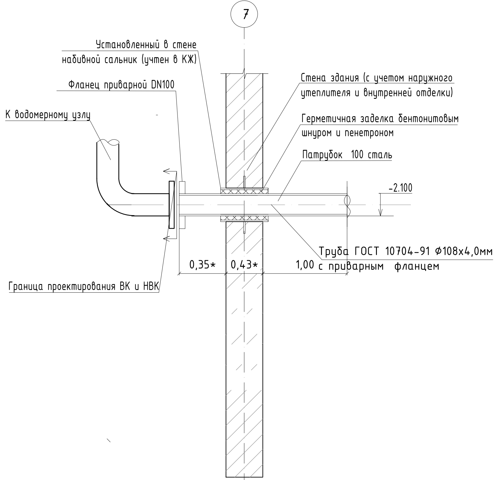
Узел прохода водопроводного ввода через фундамент
