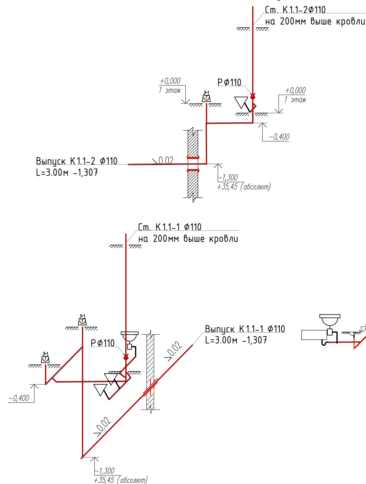
Схема водоотведения выпуск К1.1
