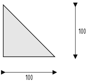
Ребро Ред-1 (48 шт) Лист t=6, сталь С245, 100×100
