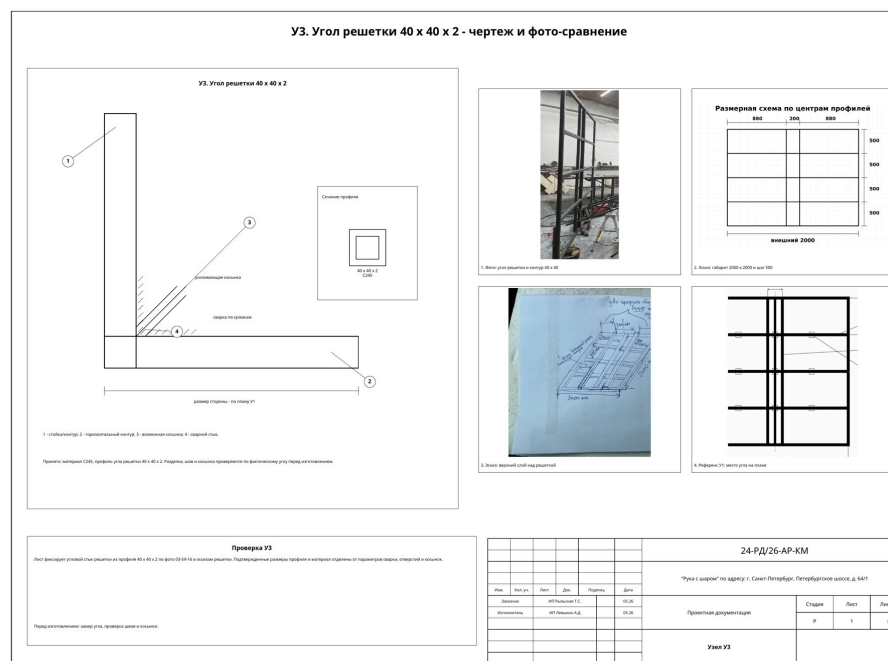
Узел УЗ: чертёж и фото ↗ • стр. 1
