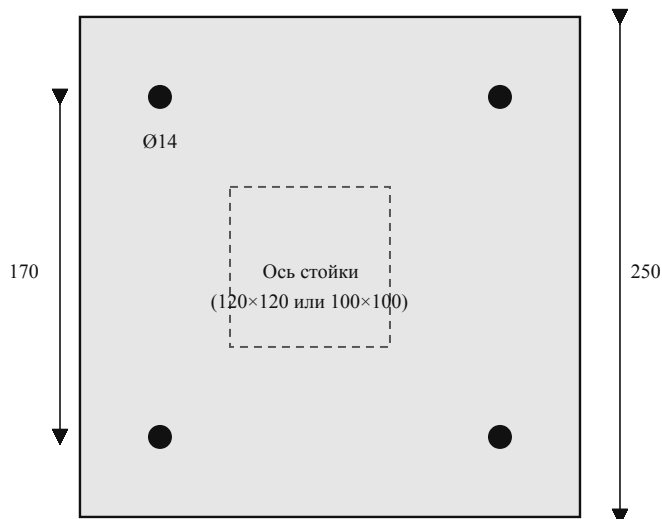
Опорная пластина ОП-1 (12 шт). Лист t=10, сталь С245, 250×250
