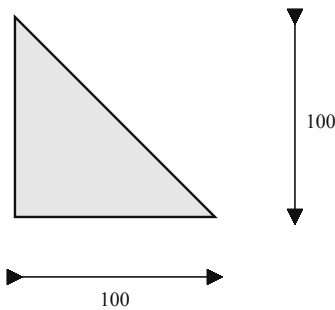
Ребро Реб-1 (48 шт) Лист t=6, сталь С245, 100×100
