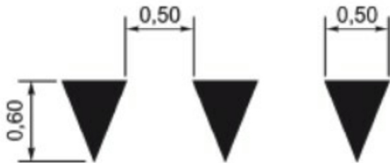
Горизонтальная разметка N1.13 по ГОСТ Р 51256–2018, цвет белый
