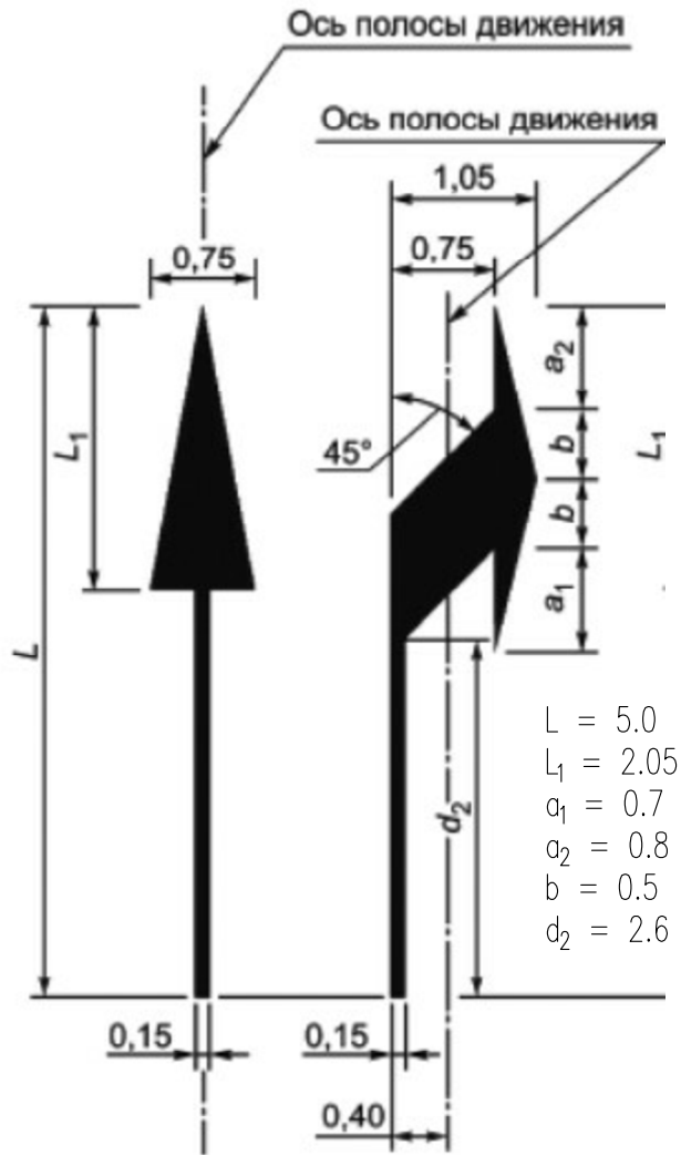
Горизонтальная разметка N1.18 по ГОСТ Р 51256–2018, цвет белый
