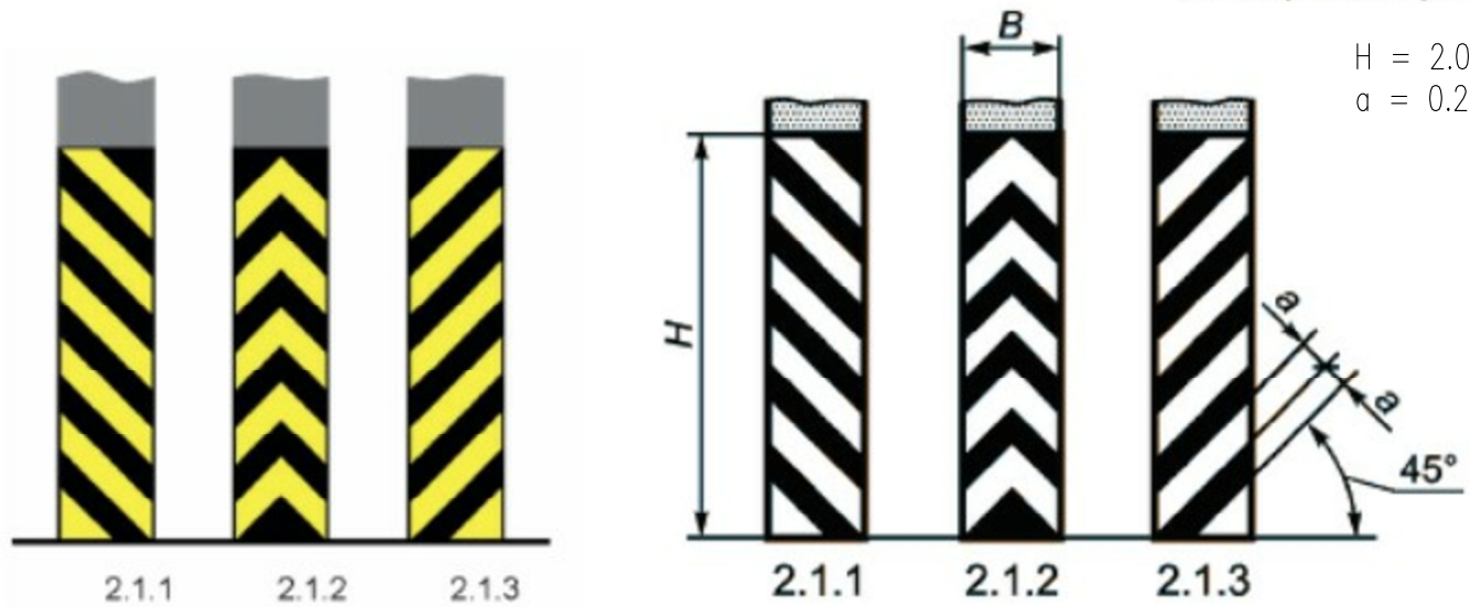
Вертикальная разметка N2.1.1–3 по ГОСТ Р 51256–2018, цвет желтый и черный
