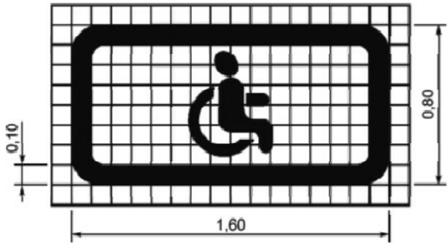
Горизонтальная разметка N1.24.3 по ГОСТ Р 51256–2018, цвет белый
