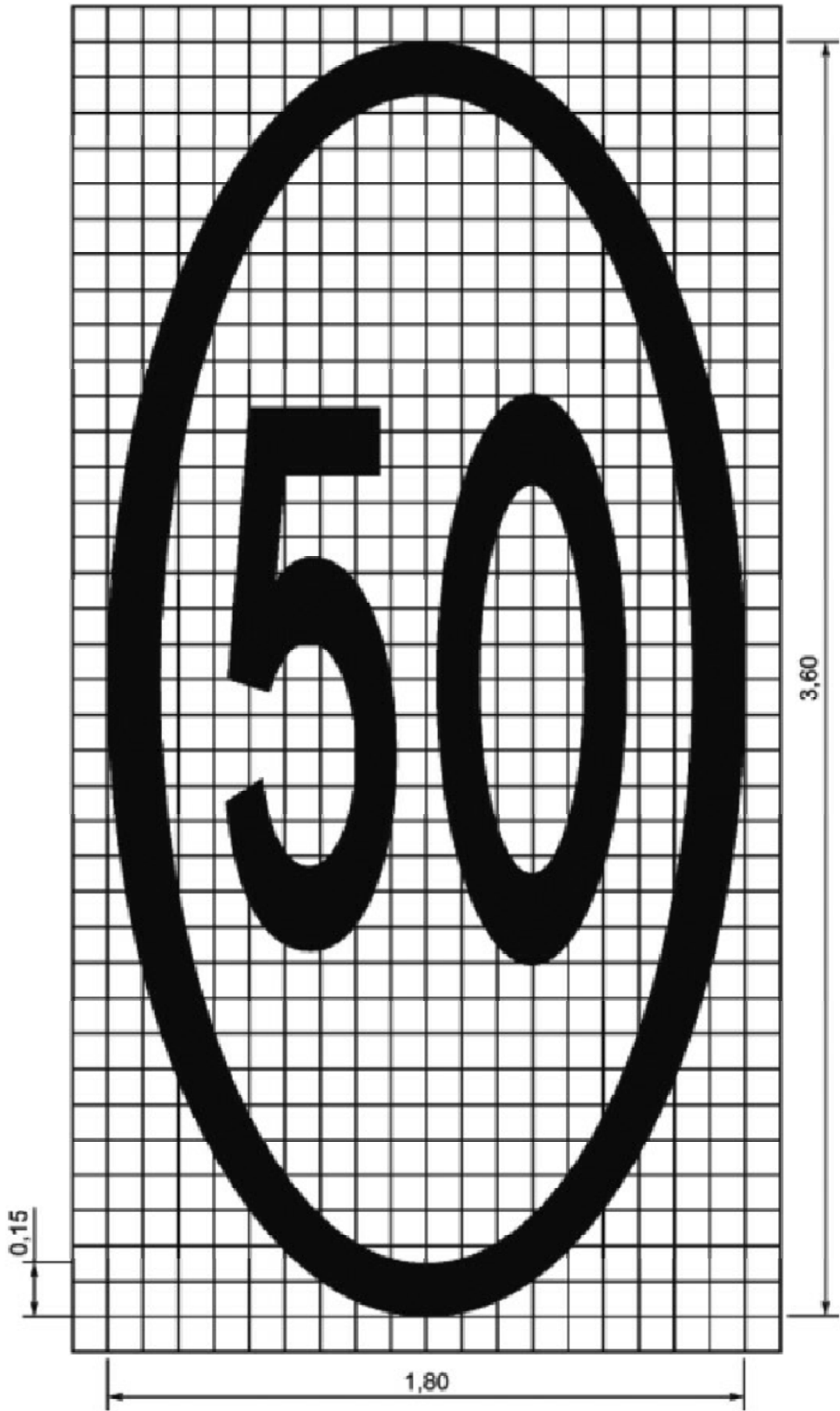
Горизонтальная разметка N1.24.2 по ГОСТ Р 51256–2018, цвет белый
